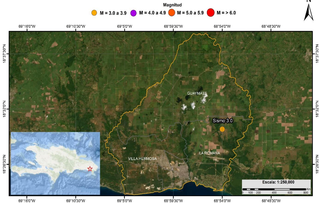
Fig. 1 Mapa epicentral
