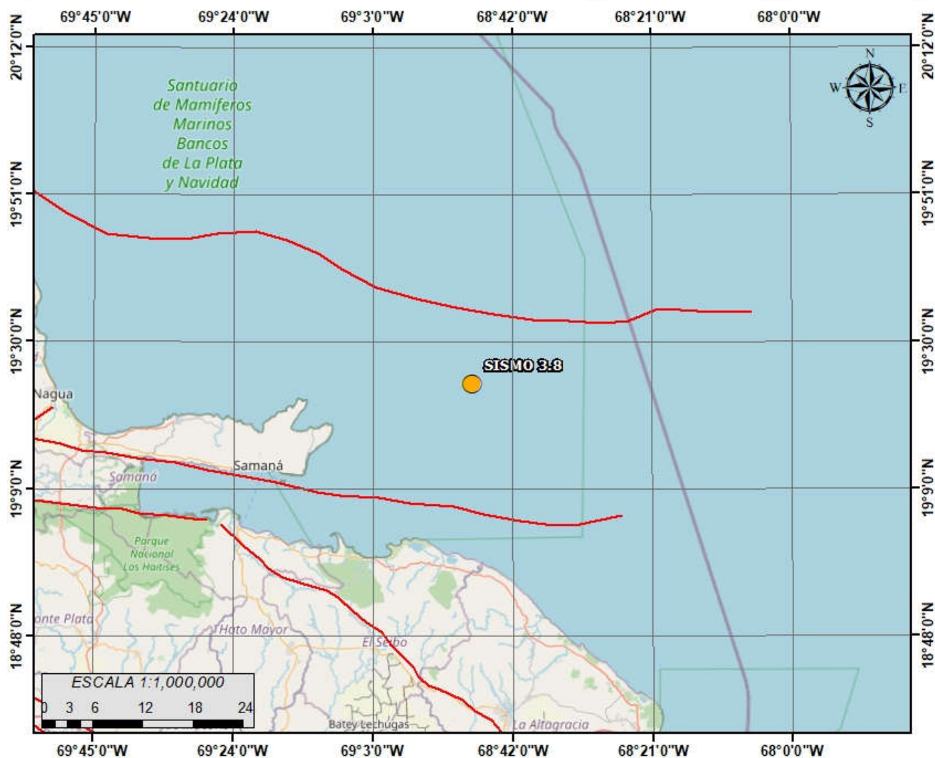
Fig. 1 Mapa epicentral
