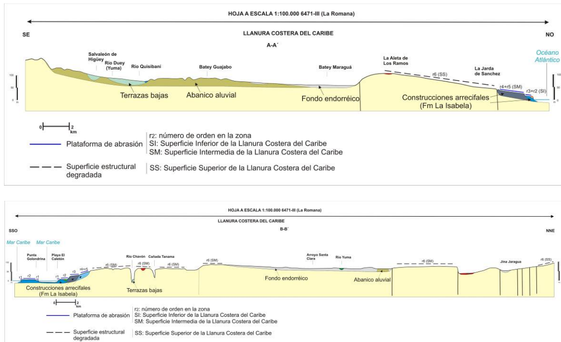
Fig. 2.2. Perfiles esquemáticos del sector oriental de la Llanura Costera del Caribe. Exageración vertical 20:1 respecto de la horizontal.
