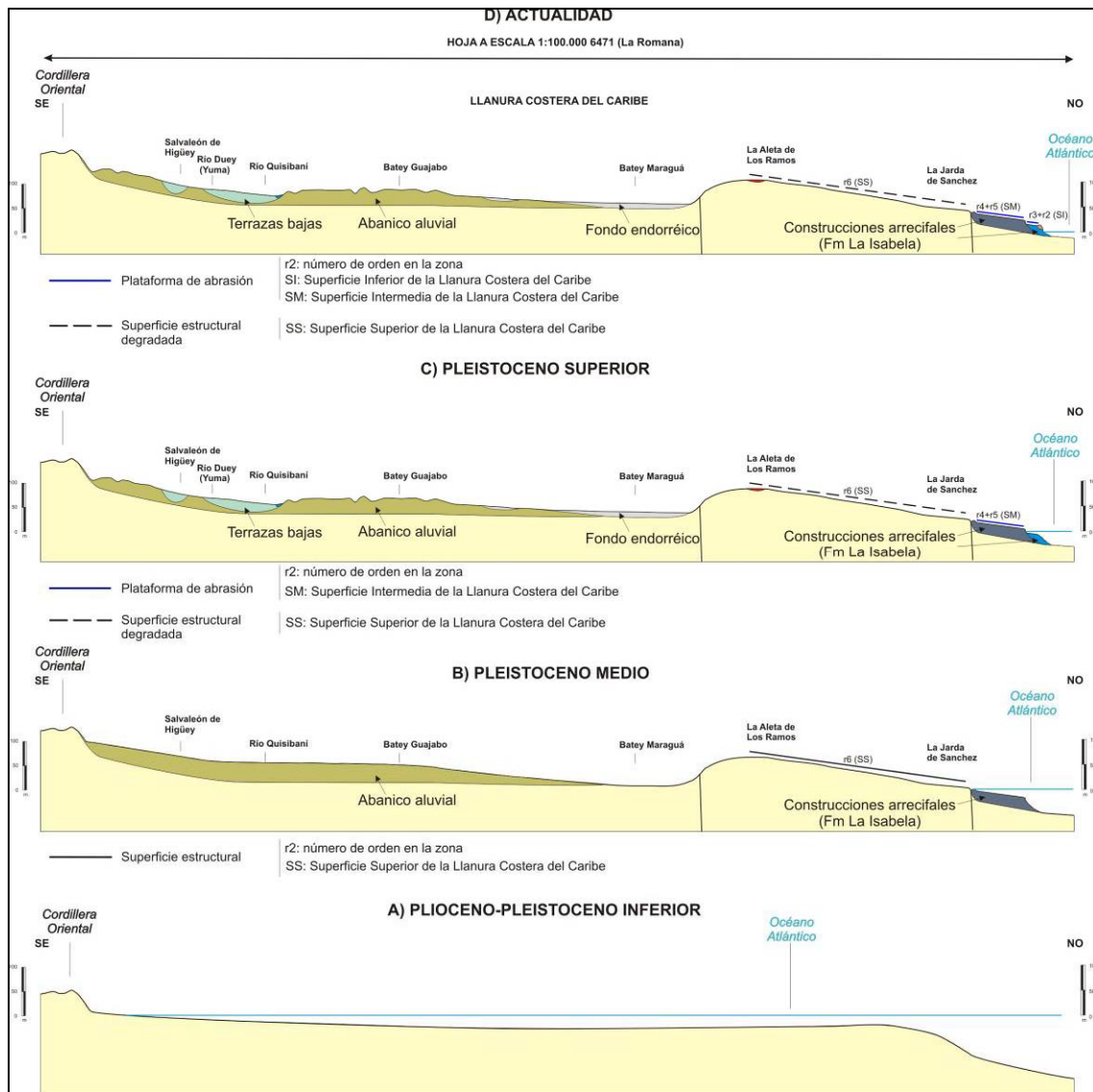
Fig. 5.2. Evolución del perfil del sector occidental de la Llanura Costera del Caribe durante el Plioceno-Pleistoceno.
