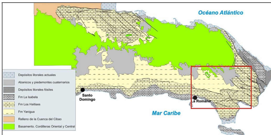
Fig.1.4. Esquema geológico del sector oriental de la República Dominicana
